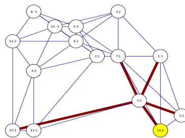
Example BFS
