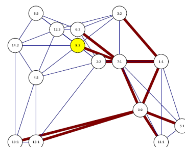
Example BFS
