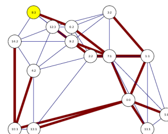
Example BFS
