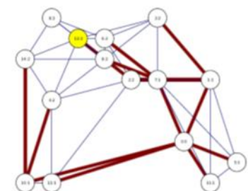
Example BFS
