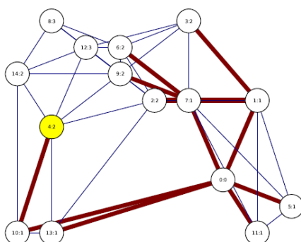
Example BFS
