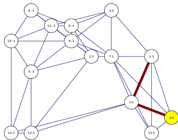
Example BFS
