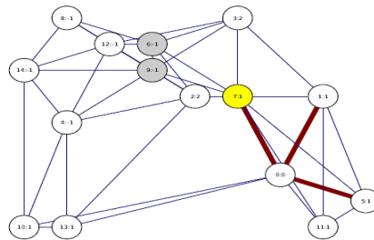
Example BFS
