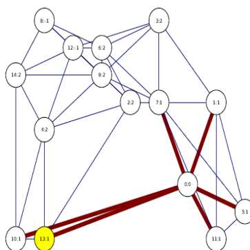
Example BFS
