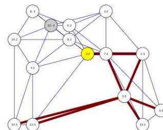
Example BFS
