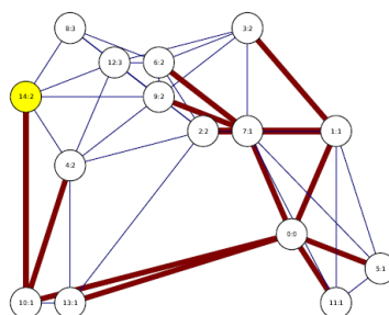
Example BFS
