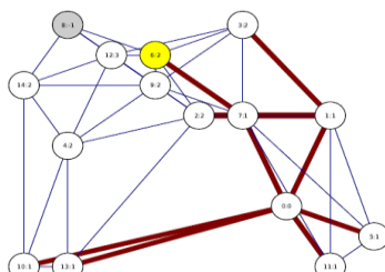
Example BFS
