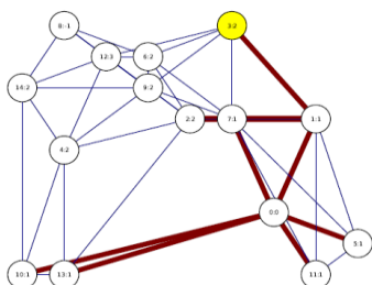
Example BFS
